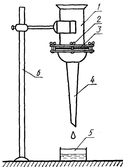
Устройство для определения показателя смачивающей способности пенообразователей
