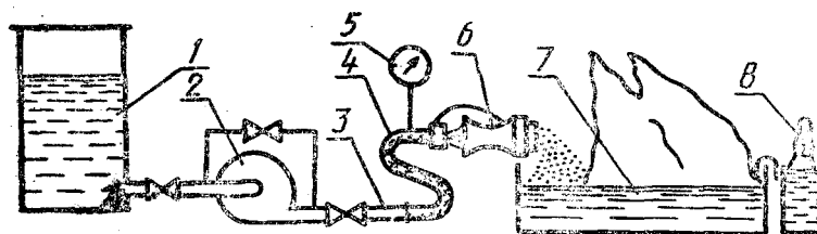
Схема установки для тушения пеной средней кратности
