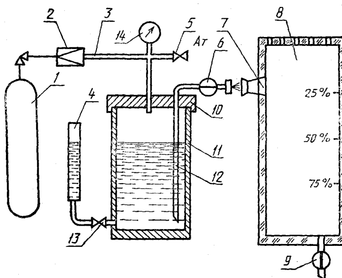
Схема установки для получения пены средней кратности
