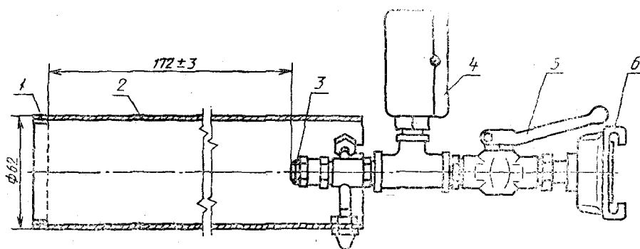
Пожарный ствол для пены средней кратности
